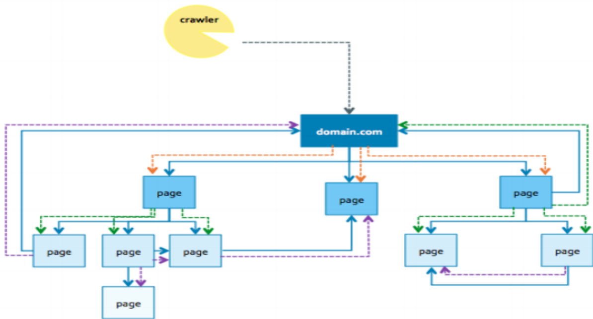
Figura 1 -Processo de arquivamento feito pelo crawler onde as linhas azuis representam os links, enquanto as linhas pontilhadas mostram o movimento de arquivamento feito pelo crawler.
